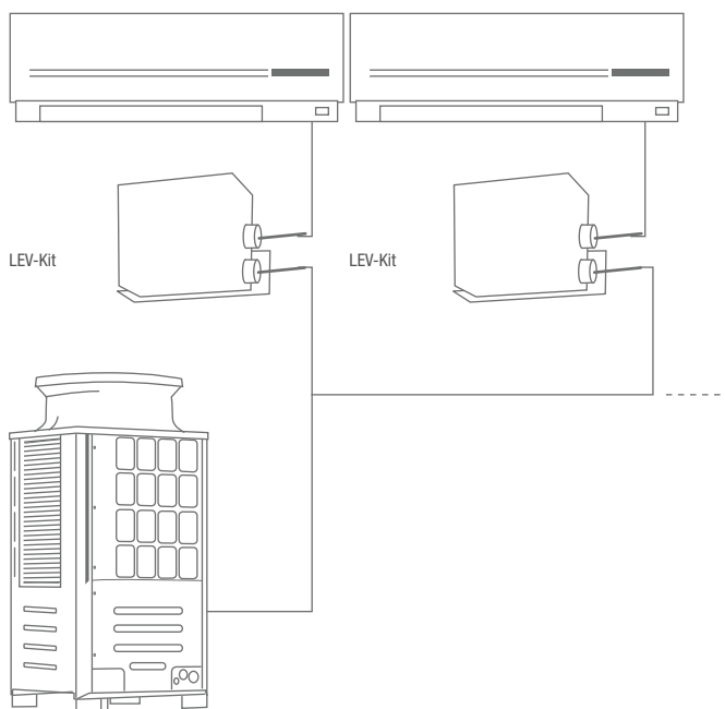
Urządzenie zewnętrzne City Multi
